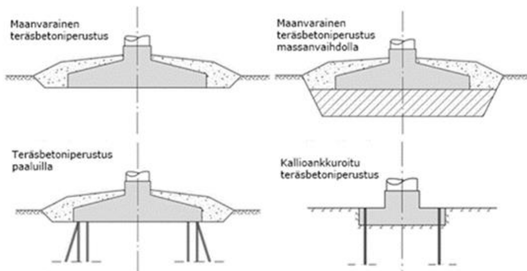
Kuva 6-2. Tuulivoimaloiden perustamistekniikoita.
